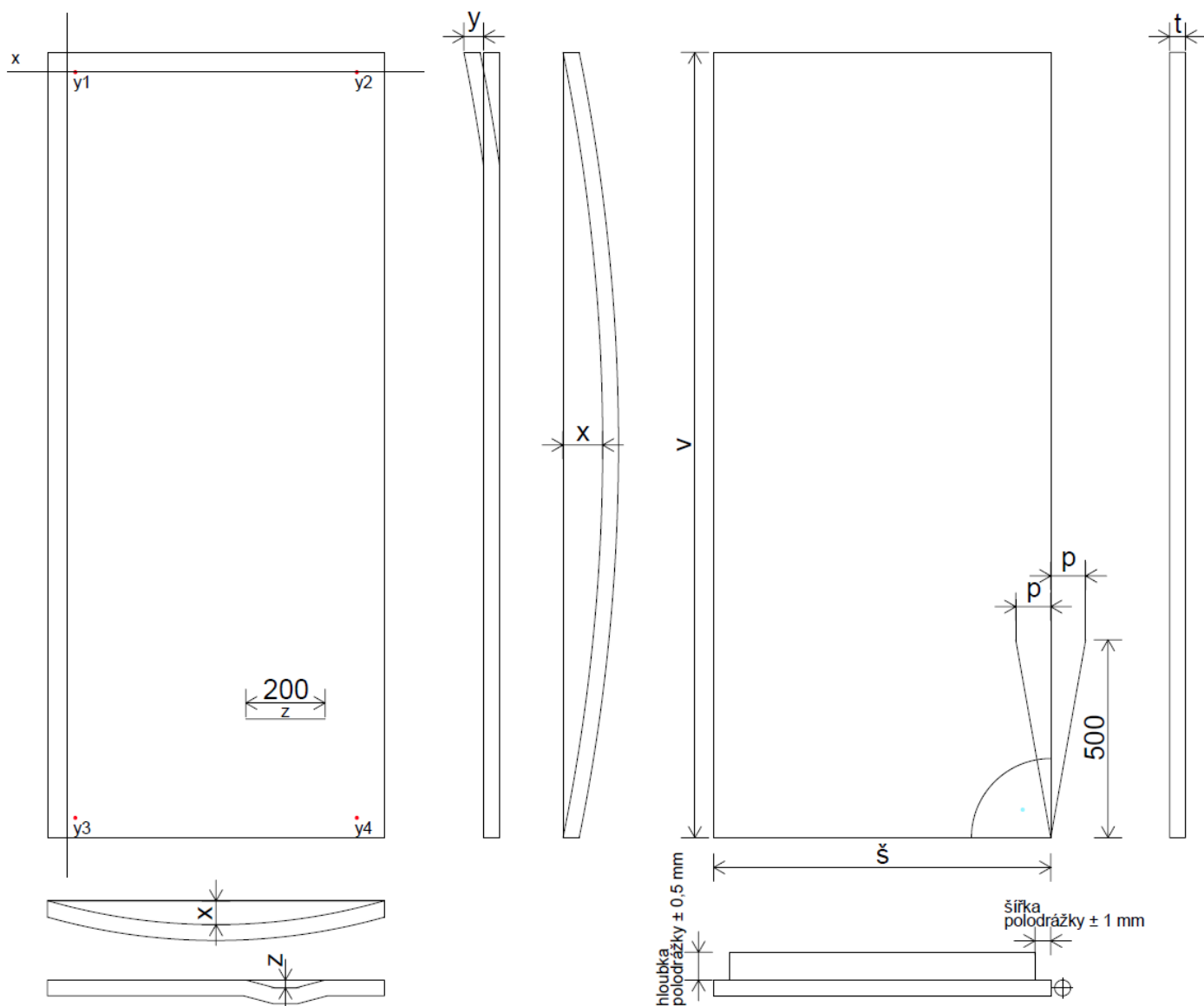
Obr.1 – Rozměrové odchylky
